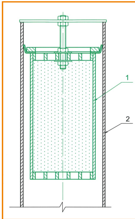
1. Geruchsdämpfungspatrone 2. Entlüftungsrohr
