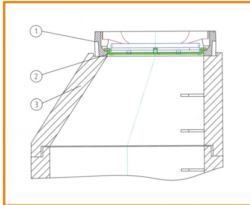
1: Schachtabdeckung mit Rahmen nach DIN 19584 2: Wasserverschluss-System FRV 3: Schacht
