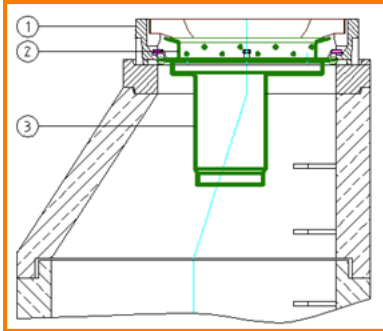
1: Schachtabdeckung mit Rahmen nach DIN 19584 2: Schmutzfang SF-3 3: Wasserverschluss-System FRK-3
